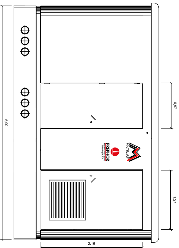
ALÇADO PRINCIPAL
