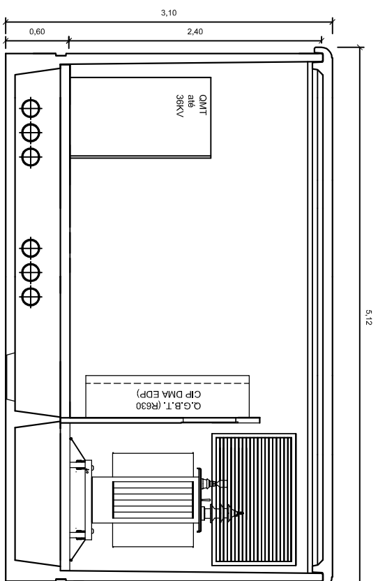
CORTE B-B'
