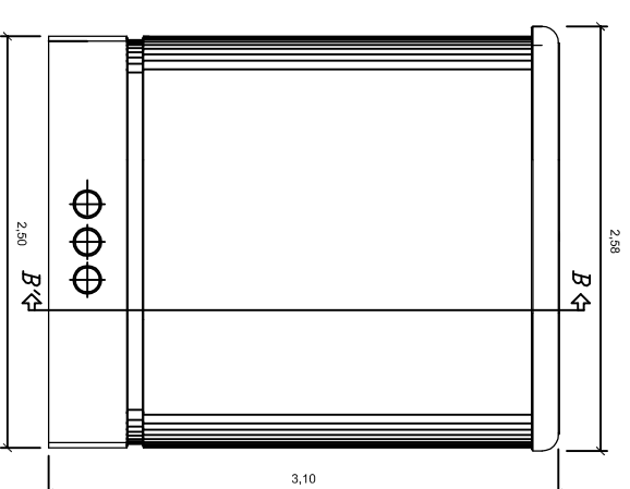
ALÇADO LATERAL ESQUERDO
