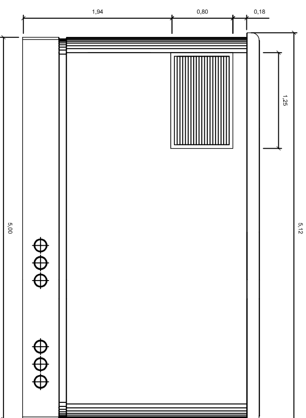
ALÇADO POSTERIOR
