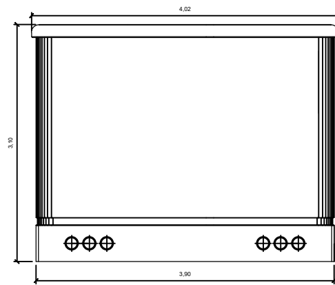
ALÇADO POSTERIOR
