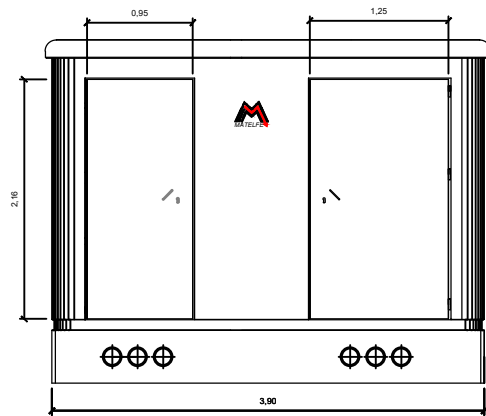
ALÇADO PRINCIPAL
