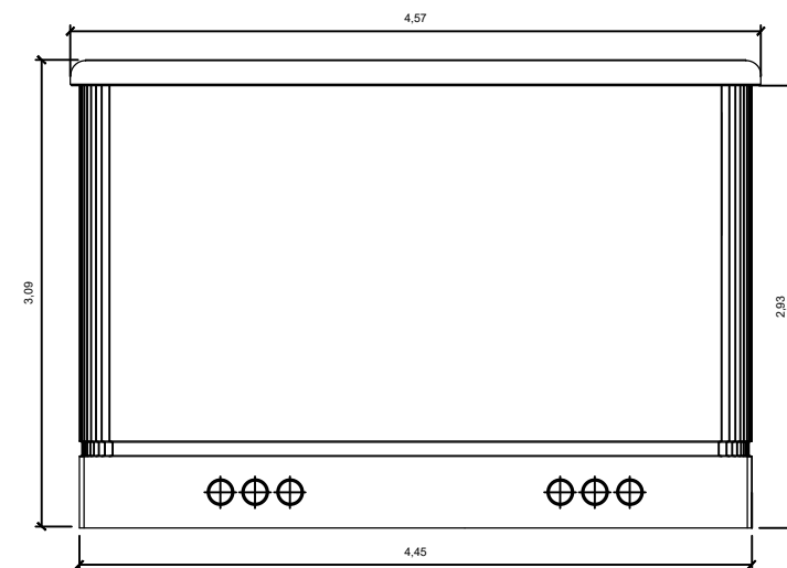
ALÇADO POSTERIOR
