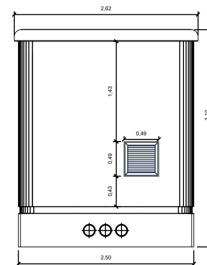
ALÇADO LATERAL DIREITA
