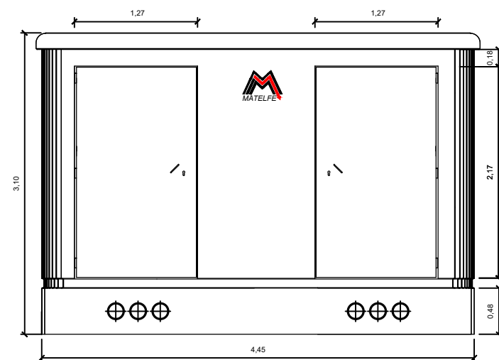
ALÇADO PRINCIPAL
