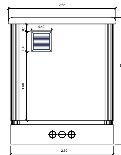
ALÇADO LATERAL ESQUERDA
