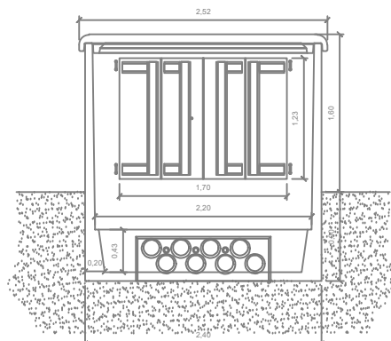
CORTE C - C'
