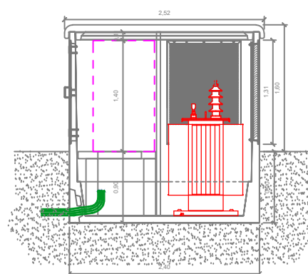
CORTE D - D'
