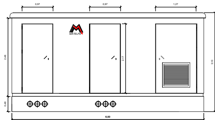
ALÇADO PRINCIPAL
