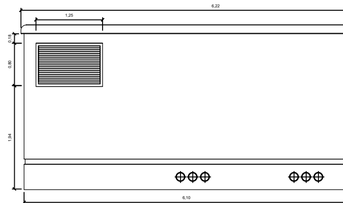
ALÇADO POSTERIOR
