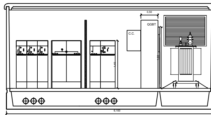
CORTE A-A'
