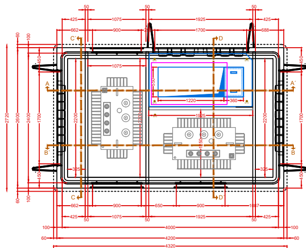
PLANTA GERAL E COTAS
