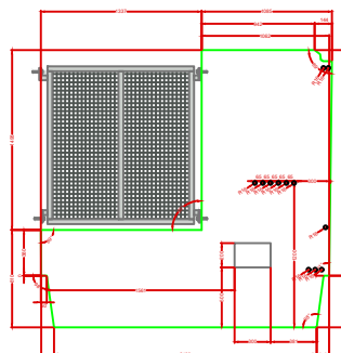
PAREDE SEPARADORA ENTRE TRANSFORMADORES
